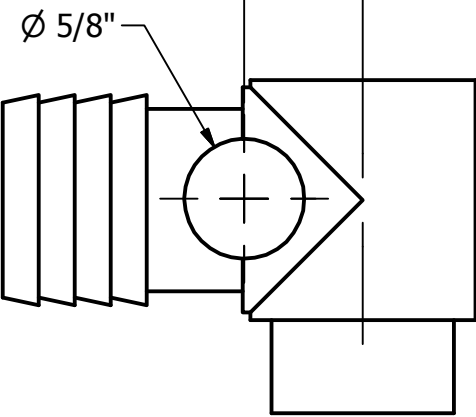
TEE à insertion en poly 1" ECHELLE 1 : 1
